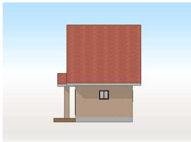
東側立面図
